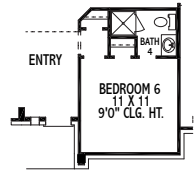
OPTIONAL BEDROOM 6 IN LIEU OF STUDY
